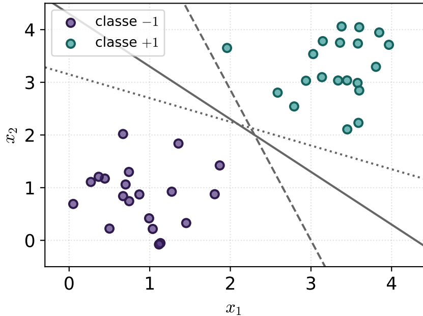
(a) Plusieurs hyperplans séparateurs
